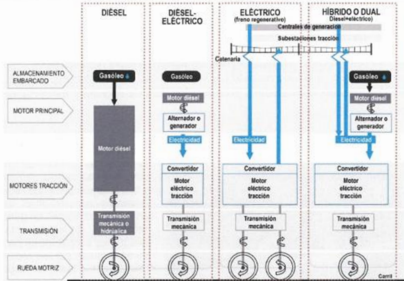
Figura 4.3. Cadena de tracción en vehículos eléctricos, diésel eléctricos e híbridos o duales (eléctrico + diésel eléctrico) LMS
