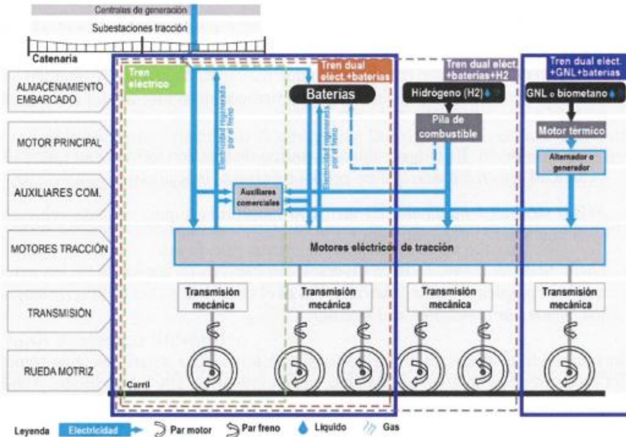
Figura 4.4. Encaje de fuentes alternativas de energía en trenes duales. LMS
