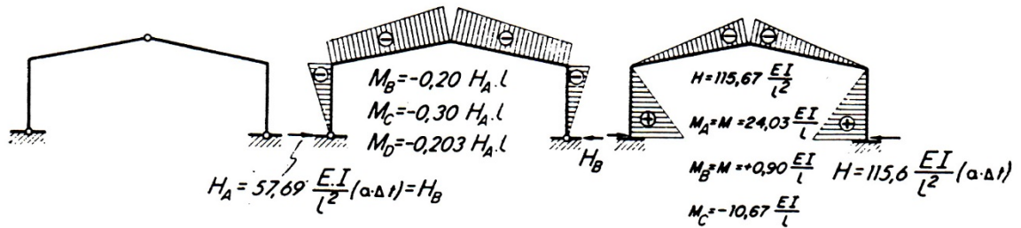
DIAGRAMA DE MOMENTOS FLECTORES Y EMPUJES DEBIDOS A UNA VARIACION DE TEMPERATURA \Delta t
