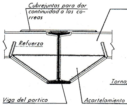
ACARTELAMIENTO DE LA CORREA
