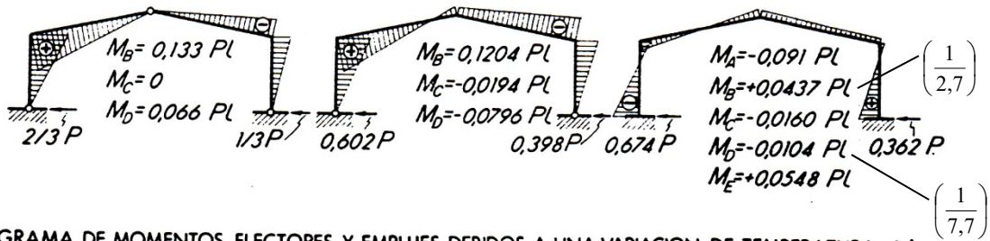
DIAGRAMA DE MOMENTOS FLECTORES Y EMPUJES DEBIDOS A UNA VARIACION DE TEMPERATURA \Delta t
