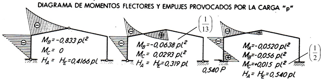
DIAGRAMA DE MOMENTOS FLECTORES Y EMPUJES DEBIDOS A LA FUERZA LATERAL "P"
