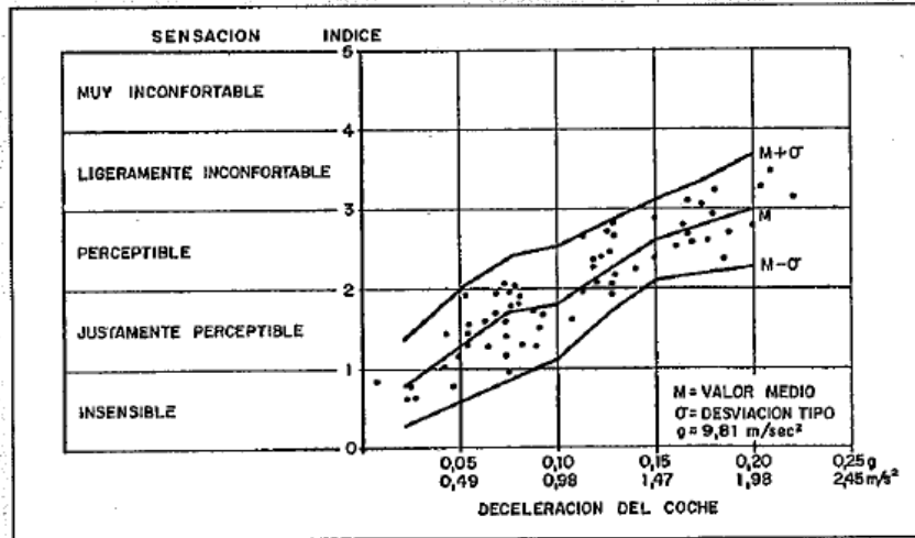
RELACIÓN ENTRE LA DECELERACIÓN DEL TREN Y EL CONFORT DE LOS VIAJEROS
