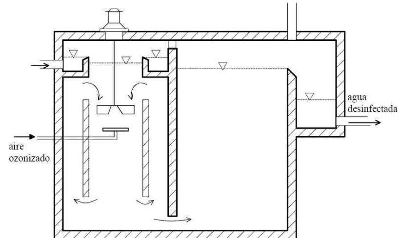
Tanque de contacto mediante turbina
