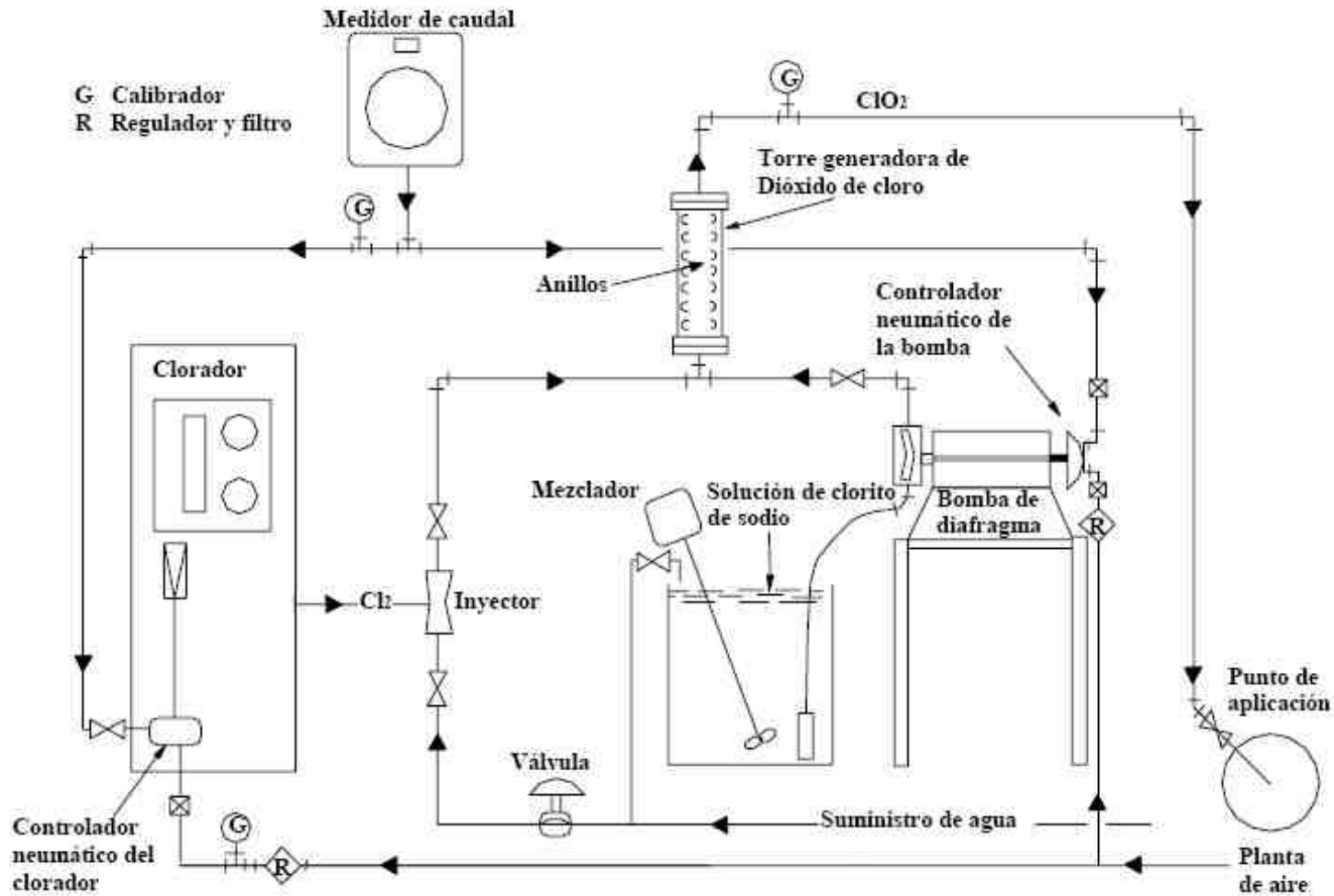
Generador de dióxido de cloro con un sistema de dos componentes
