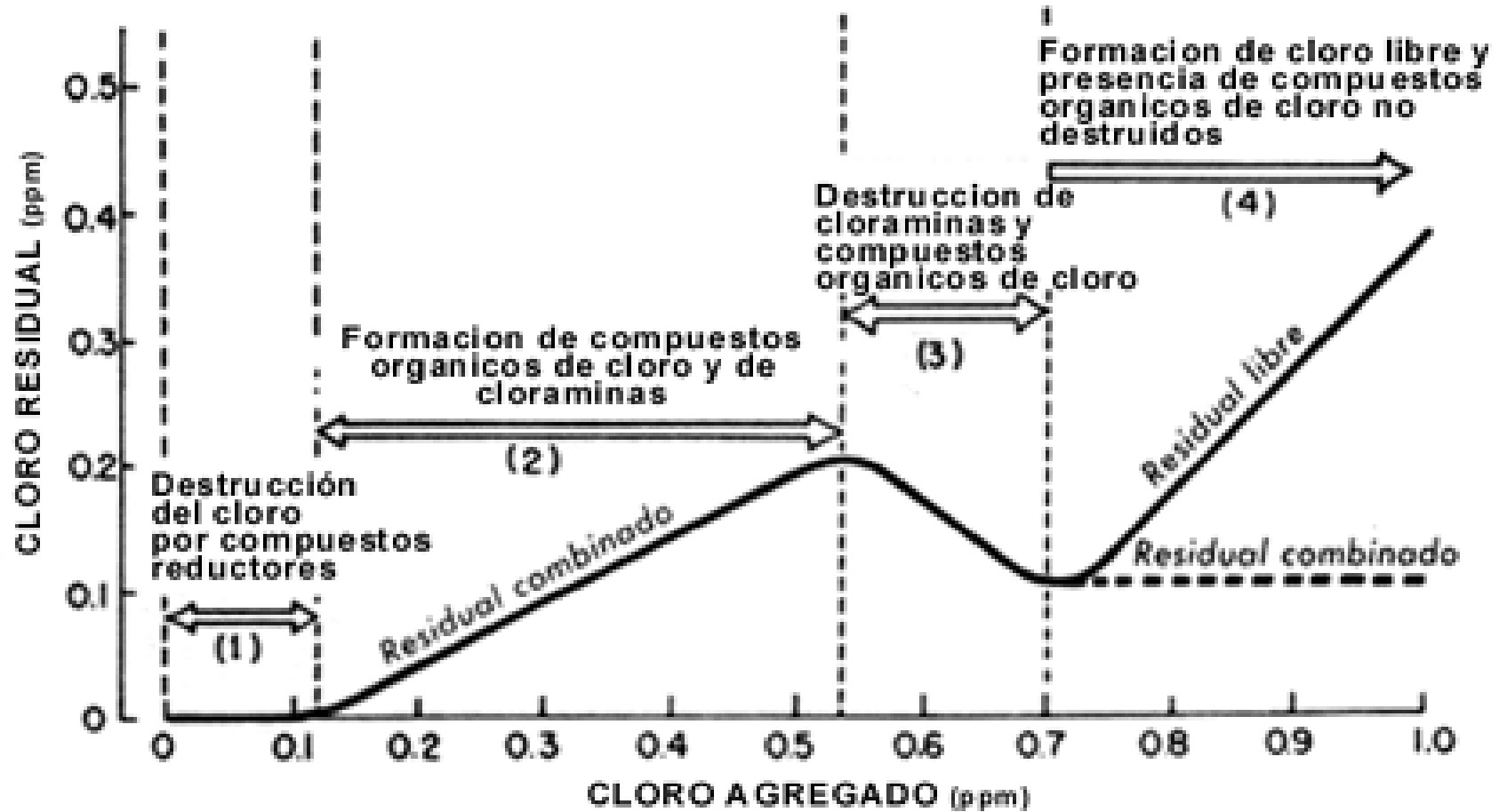
Curva de demanda de cloro (Hernández, 2001)
