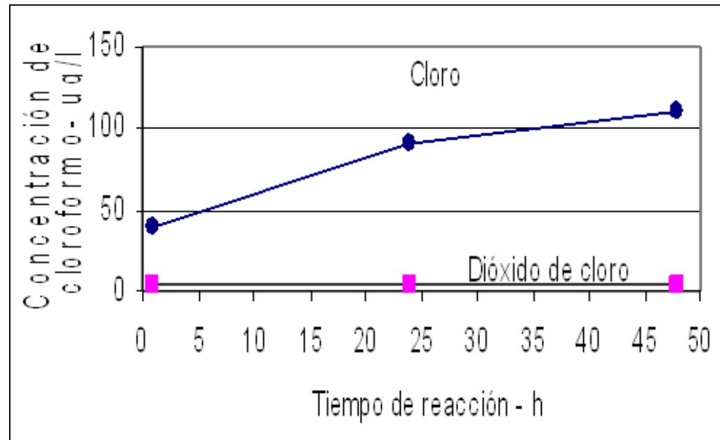
Comparación en la formación de THL por tratamientos de cloro y dióxido de cloro
