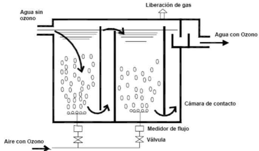
Tanque de contacto de cámara con difusores
