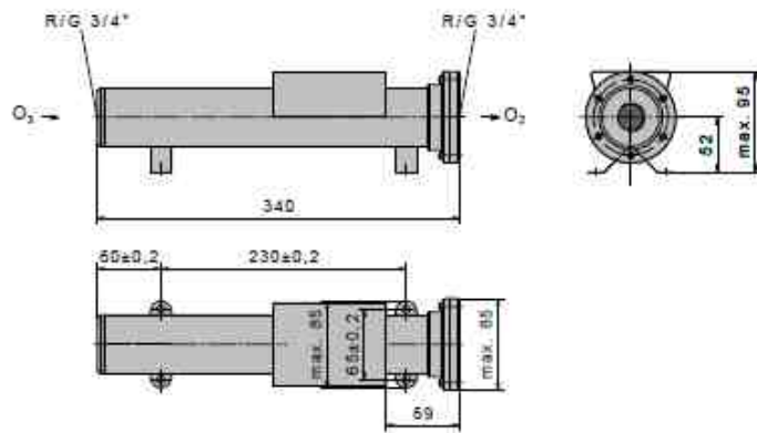
Destructor catalítico de ozono KVM Innovatec
