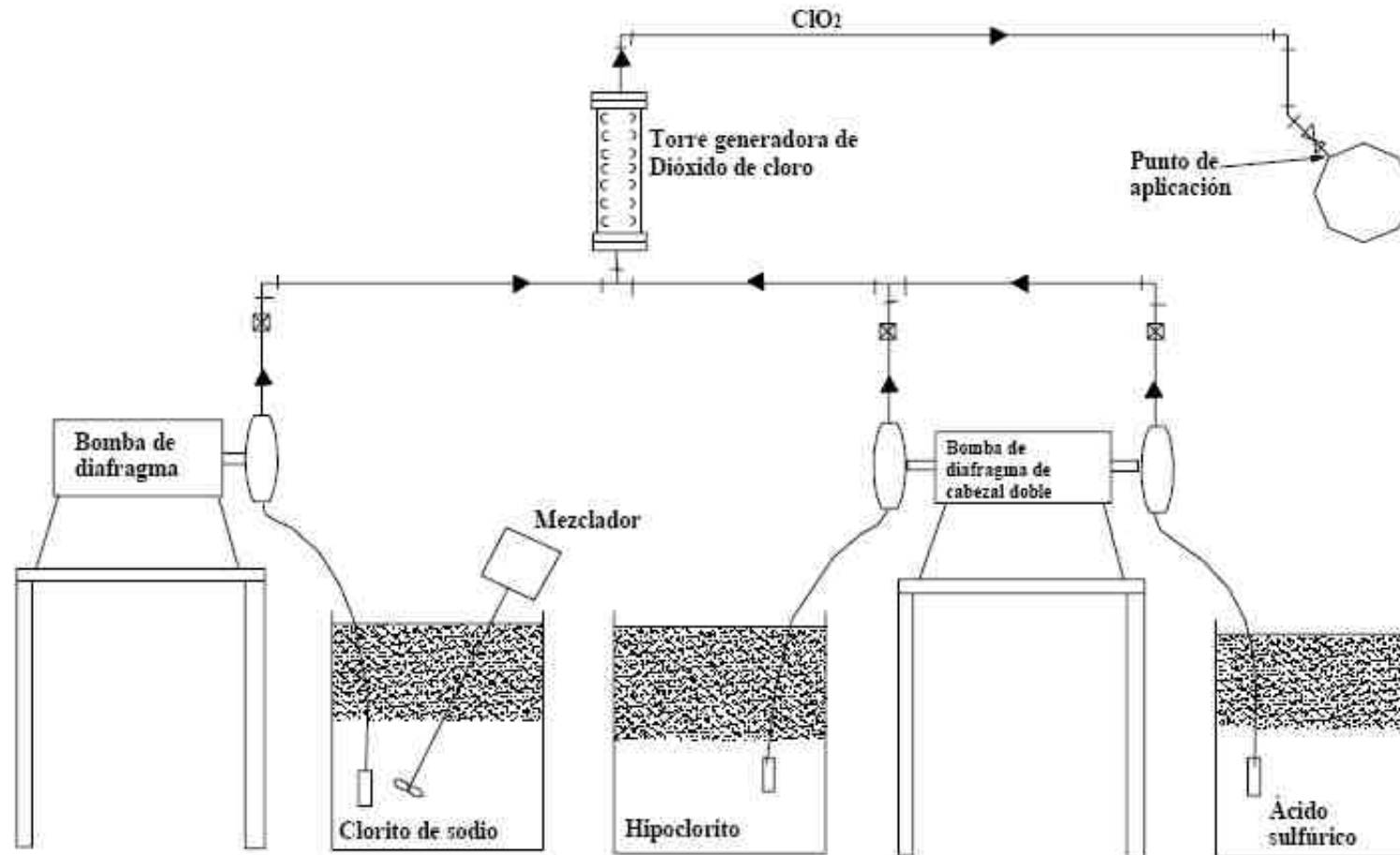
Generador de dióxido de cloro con un sistema de tres componentes
