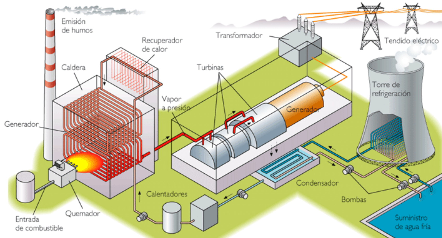
Esquema de una central térmica
