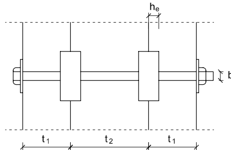
Figura 8.13 Espesores mínimos de las piezas.
